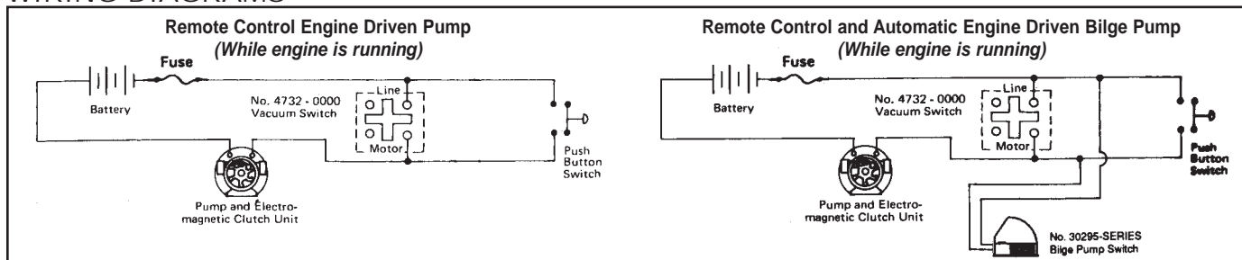
WIRING DIAGRAMS
